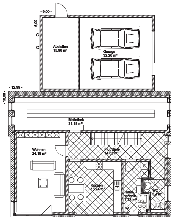
Erdgeschoss
