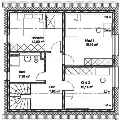
Dachgeschoss
